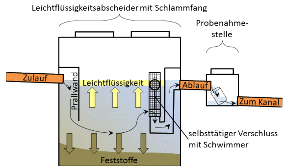
Abbildung 1: Schema eines Leichtflüssigkeitsabscheiders mit Probenahmestelle (Seitenansicht)
